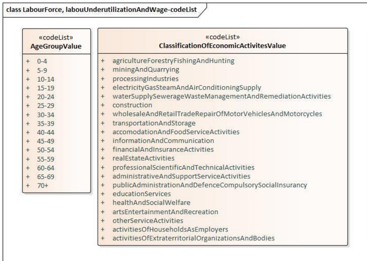
С.6-р зураг - UML диаграмм: Хөдөлмөр эрхлэлт, хөдөлмөрийн дутуу ашиглалт, дундаж цалин багцын кодын жагсаалт
