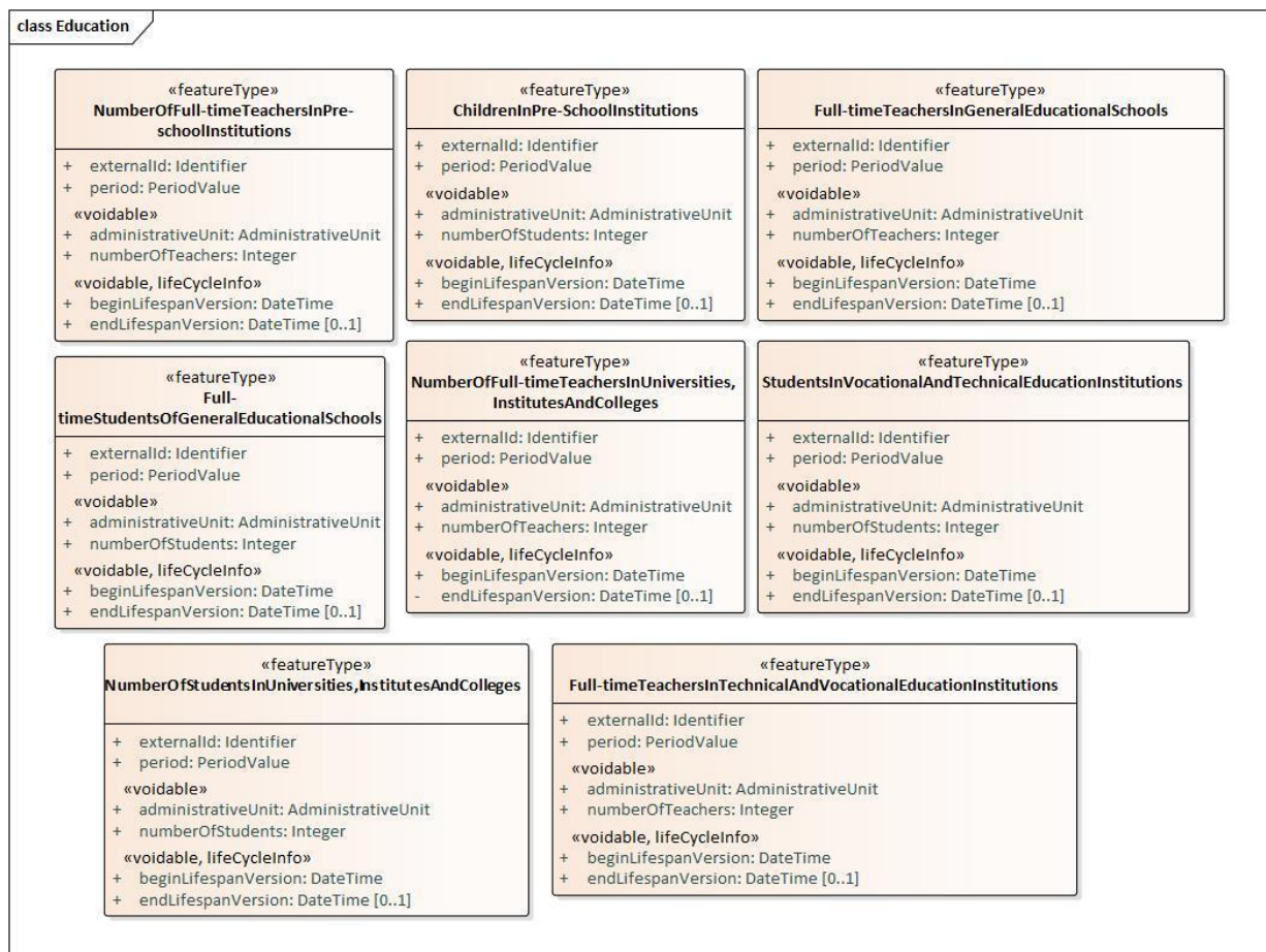
C.11-р зураг - UML диаграмм: Боловсрол багцын ерөнхий хүснэгт
