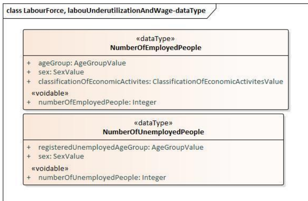
C.5-р зураг - UML диаграмм: Хөдөлмөр эрхлэлт, хөдөлмөрийн дутуу ашиглалт, дундаж цалин багцын өгөгдөл төрөл
