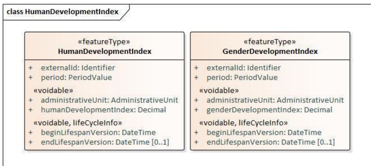
C.11-р зураг - UML диаграмм: Хүний хөгжлийн индекс багцын ерөнхий хүснэгт
